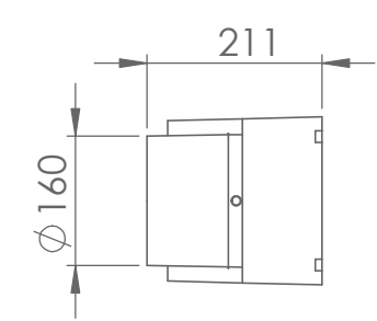
euromatic Luftklasten (Darstellung ohne Luftgitter)
