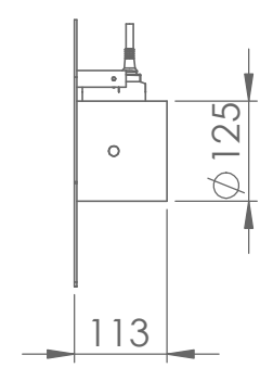
euromatic Aussenluftadapter senkrecht
